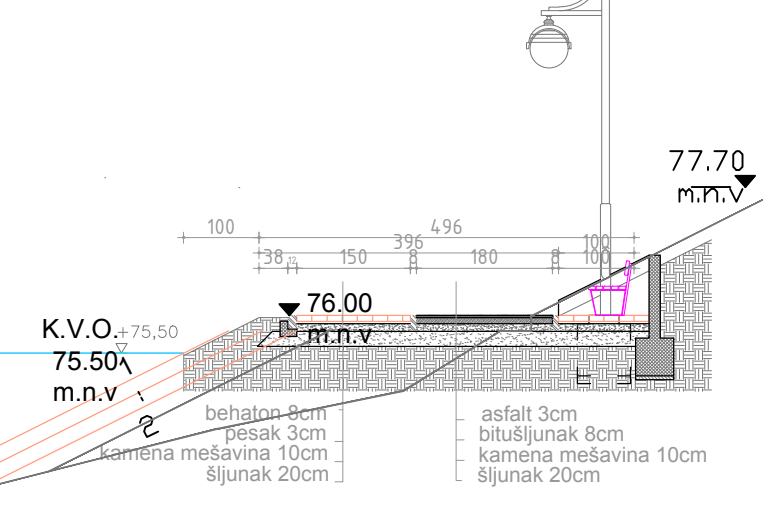
ПРЕСЕК 1-1 P-1:100
