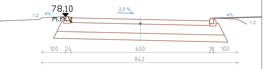
ПРЕСЕК 3-3 P-1:100
