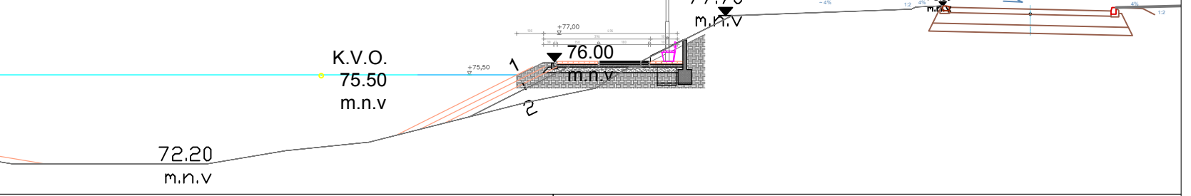
ПРЕСЕК 1-1 P-1:100
