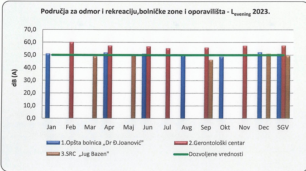
Grafik br. 2 Indikator večernje buke
