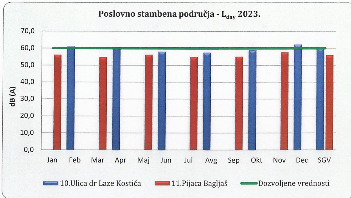
Grafik br. 13 Indikator dnevne buke
