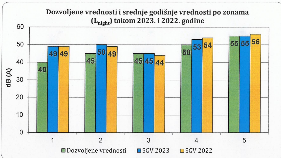
Grafik br. 23 Dozvoljene vrednosti i (SGV)-noćni intervali merenja tokom 2023. i 2022. godine
