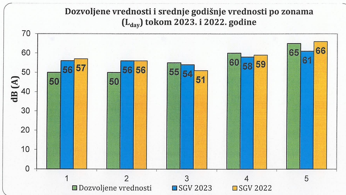
Grafik br. 21 Dozvoljene vrednosti i (SGV)-dnevni intervali merenja tokom 2023. i 2022. godine
